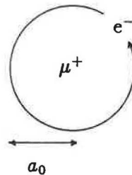
Muonium
